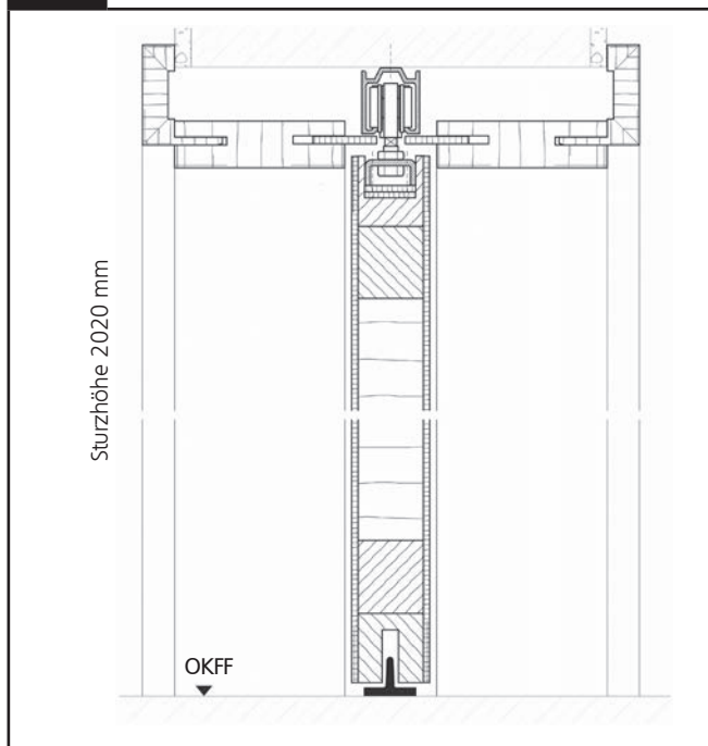
Schiebetür unter Sturz
