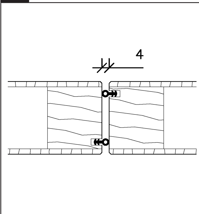
Anschluss bei 2-flügeligen Türen
